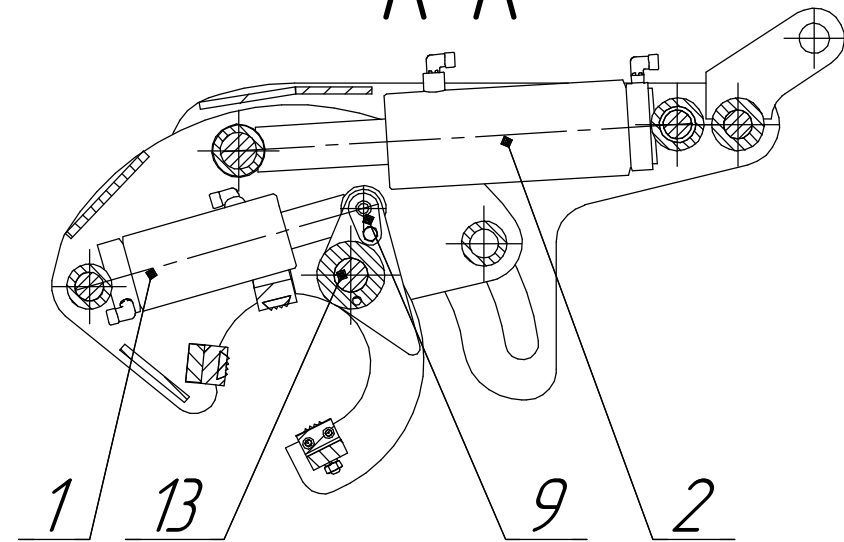
A-A
