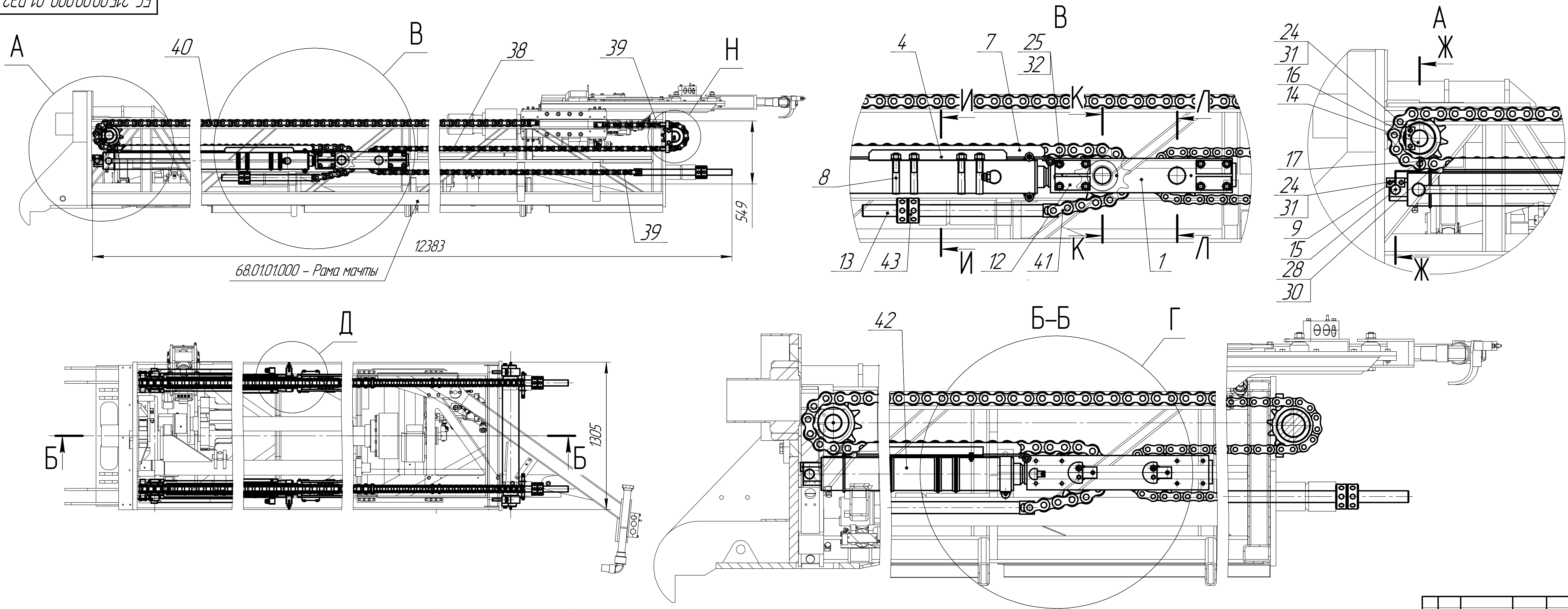
Рисунок 2.9 Механизм подачи 68.0109.000
