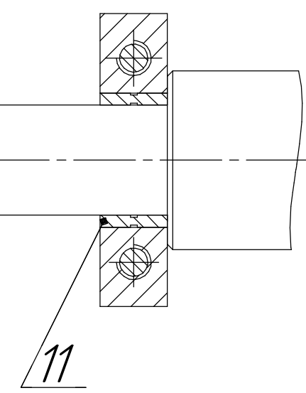
Б-Б
