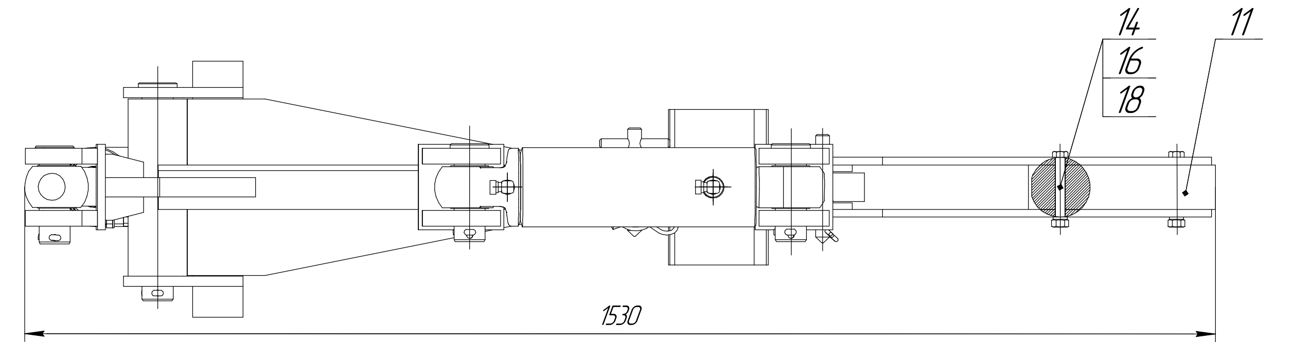
Рисунок 2.6 Люнет 68.01.05.000
