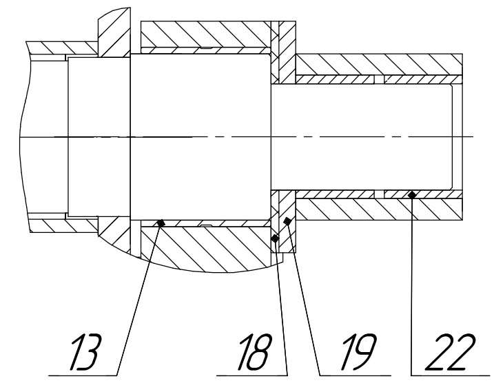
Рисунок 2.5 Механизм поворота штанг 68.01.03.000
