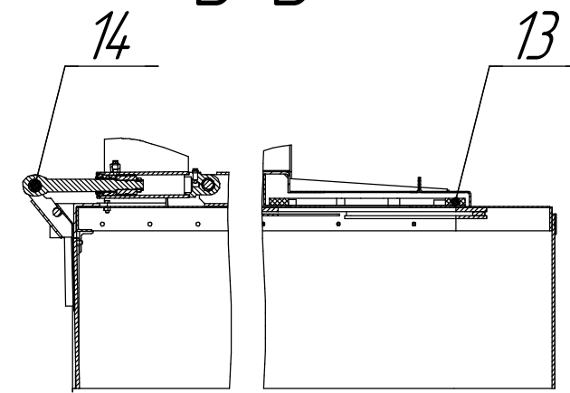
В-В
