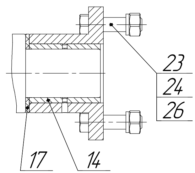
Д-Д(1:4)
