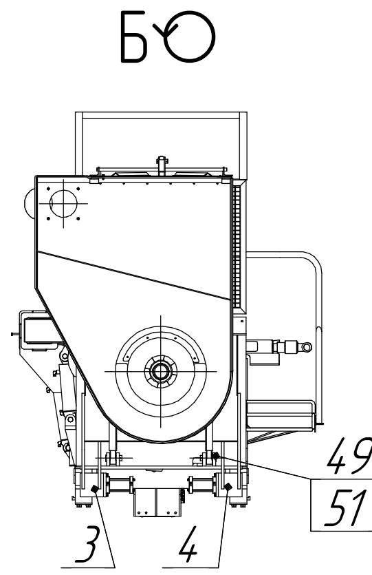
Рисунок 2.4 Мачта 68.01.00.000
