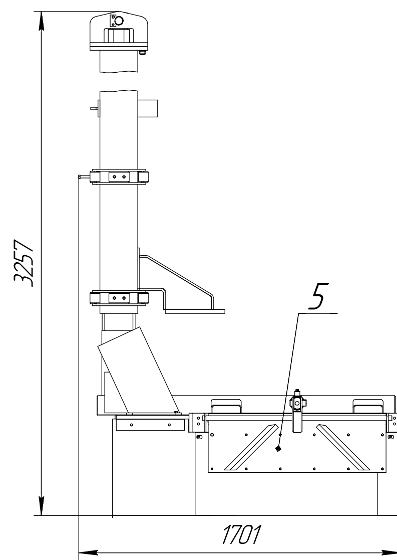
Б-Б
